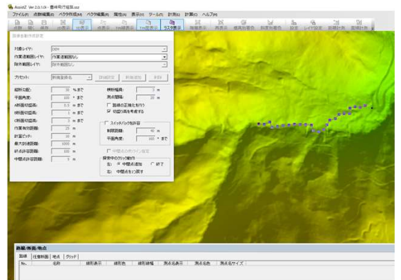
図2 林内作業道開設シミュレーター
